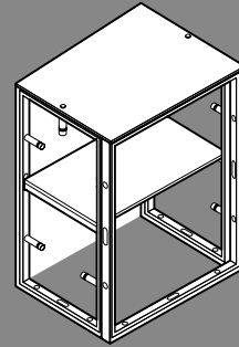
Clever Frame technical counter / Clever Frame technischer Theke
